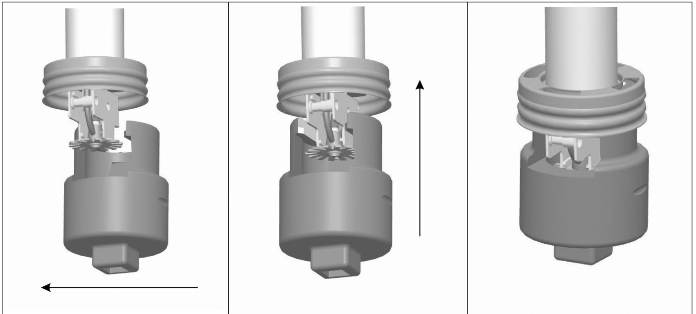
Fig. 13 - Model XLO2 Wrench
